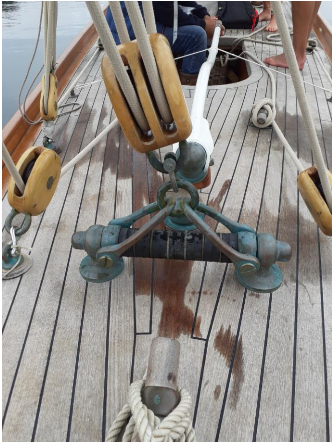
Détail du point d'amure de l'écoute de grand voile avec son amortisseur
