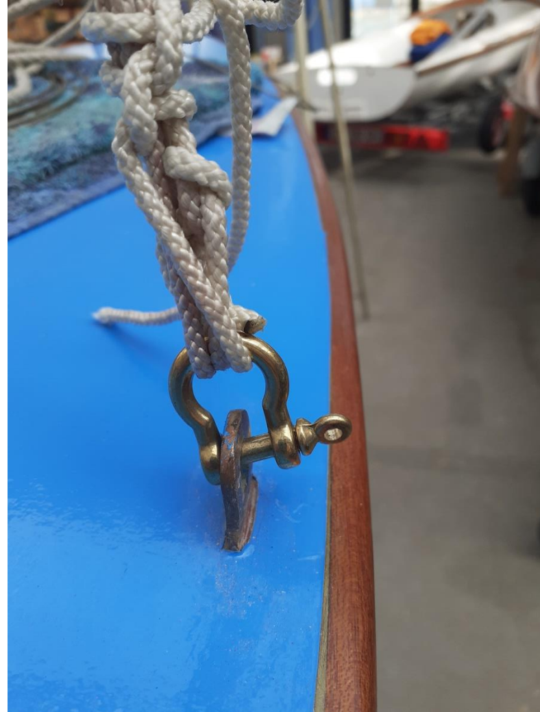
Détails de fixation des haubans avec manille bronze
