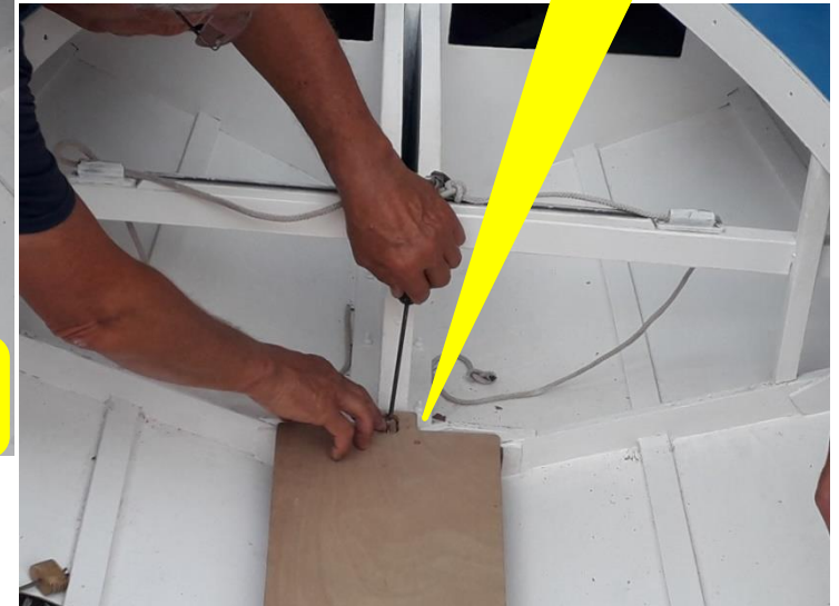
Détail de fixation avant du couvre quille
